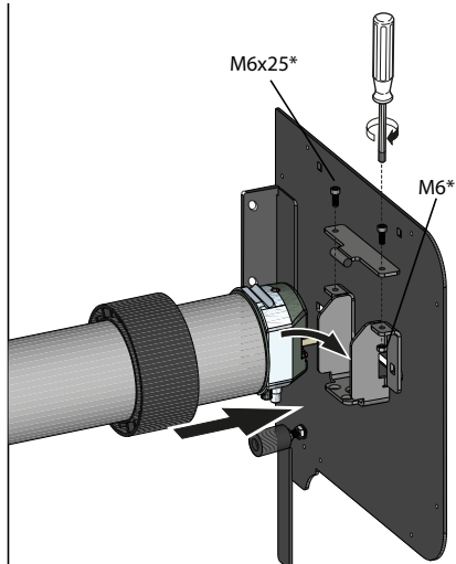
MOTOR SERIE 8 MMS
