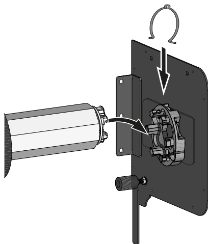
MOTOR SERIE 6 STD
